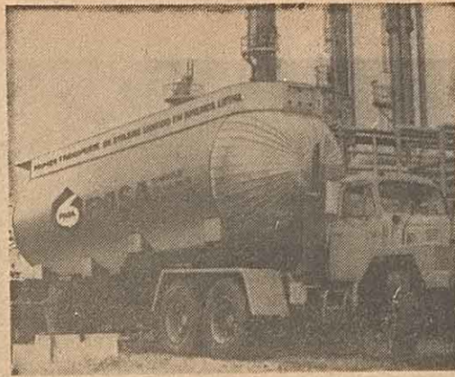
En este camión, construido por la industria nacional, que cuenta con especialísimas condiciones, se transporta el etileno líquido.
