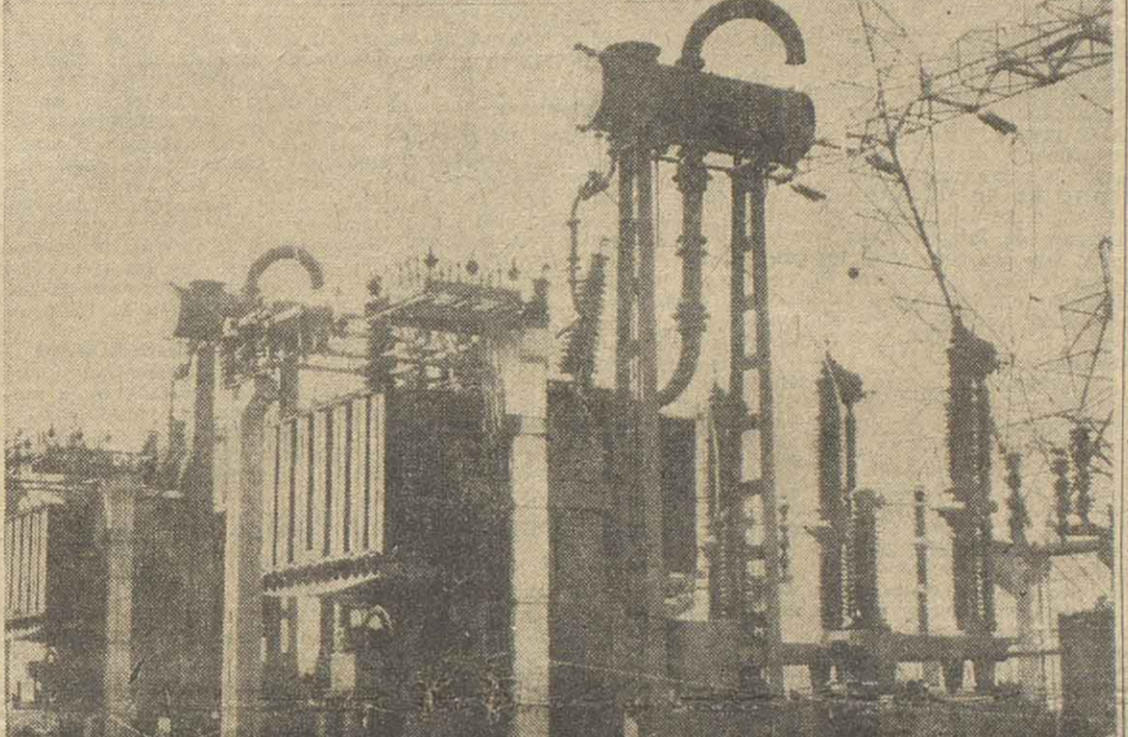
Los enormes transformadores de 26.000 kilovatios cada uno, instalados en la estación sur de nuestra ciudad y destinados a la reducción a 13.000 voltios de tensión a que viene la corriente enviada desde San Nicolás a nuestra ciudad. Con esta obra, y otras que se están llevando a cabo quedará solucionado definitivamente el grave problema energético de Rosario.
